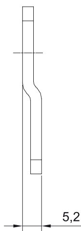
Schließhebel Variante 3 Locking lever option 3
